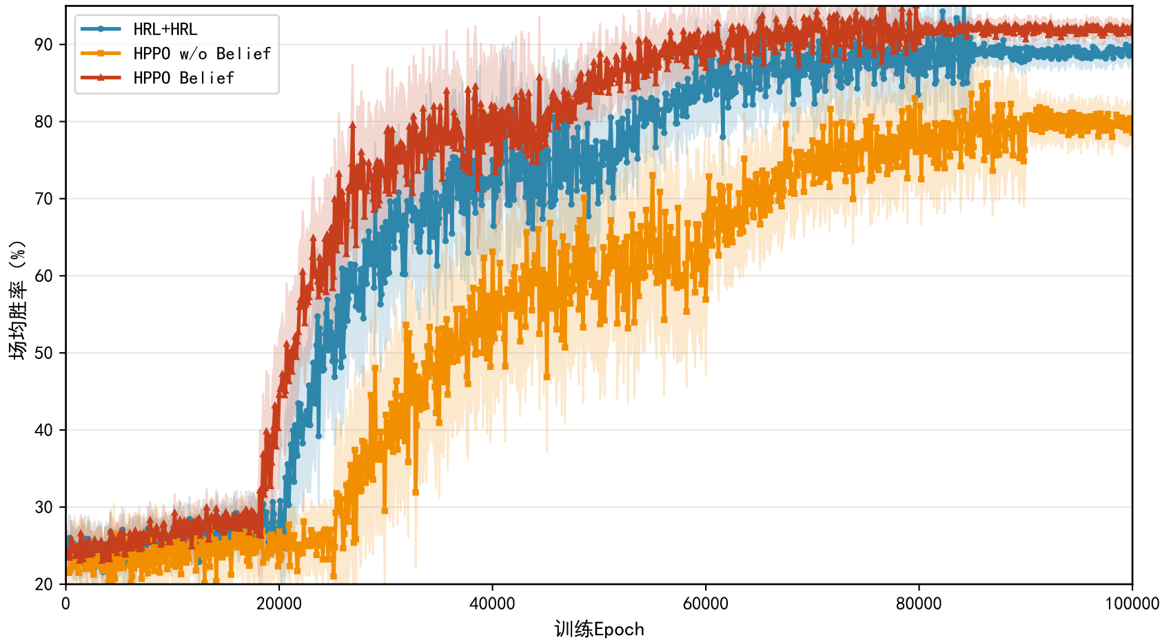
多模型训练胜率收敛曲线对比（对战RuleRobot+RuleRobot）
